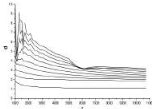
Gambar 3. Grafik hubungan dimensi korelasi dan r tremor vulkanik menunjukkan scaling region di sekitar r=5500-6500 dan d=3,14
