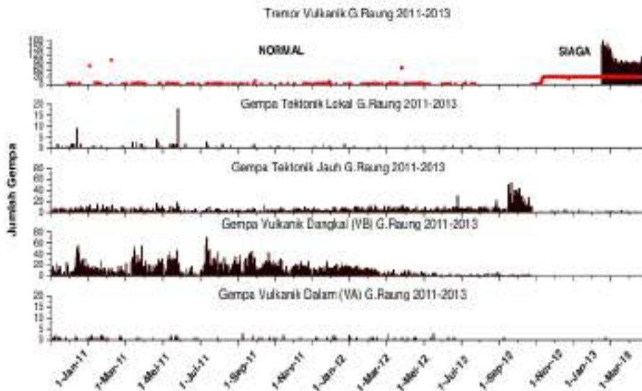
Gambar 4. Aktifitas kegempaan gunung Raung
