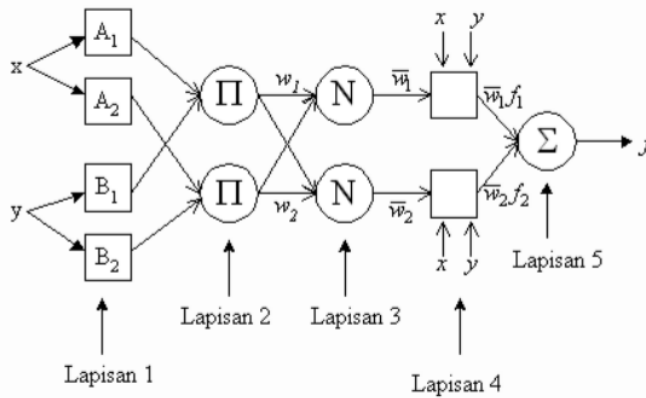
Gambar 1. Arsitektur ANFIS
