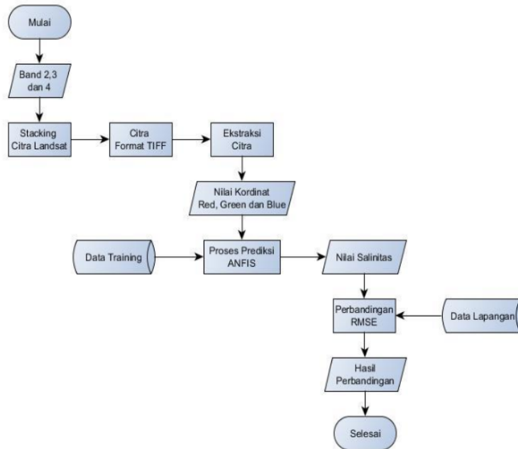
Gambar 2. Flowchart proses analisa data, perancangan, pembangunan dan pengujian sistem
