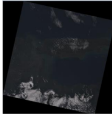
Gambar 3. Hasil Stacking band 2,3 dan 4
