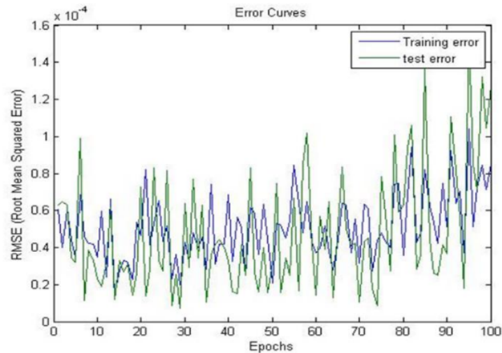
Gambar 3. pengukuran error antara training data dan testing data menggunakan RMSE
