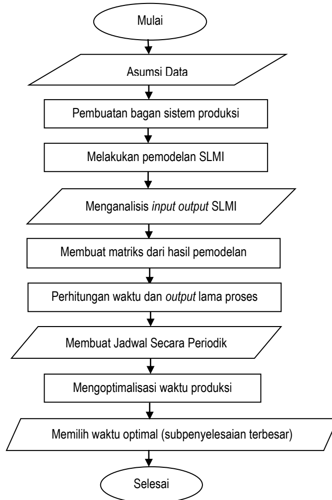
Gambar 2. Diagram Alir Metode SLMI pada Aljabar max-Plus
