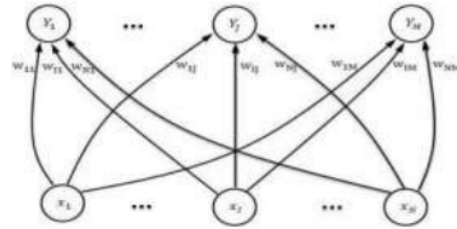
Gambar 1 Struktur Jaringan Syaraf Tiruan Kohonen SOM
